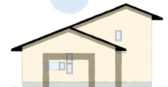
東側立面図
